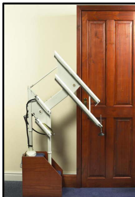
VOLLAUTOMATISCHE EINSCHUBSCHIENE
